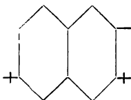
R Säure. D.R.P. 3229.
